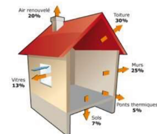
Perte de chaleur d'une maison individuelle non isolée
